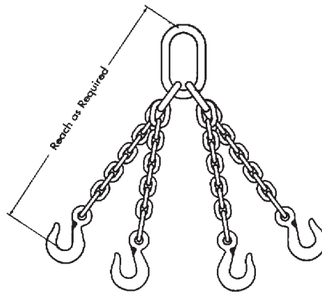
Type QOS
