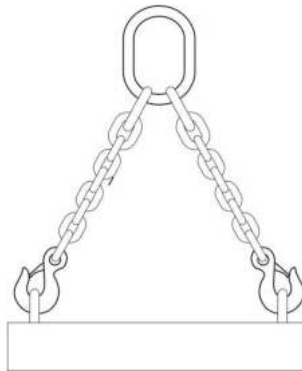
(d) Double-Leg Bridle Sling Hitch
