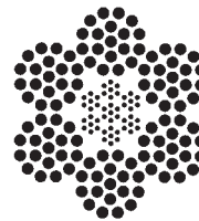
6x19 IWRC
